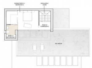
PLANTA ALTA / TOP FLOOR
