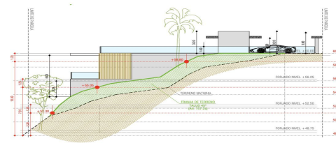
ALZADO NORTE
